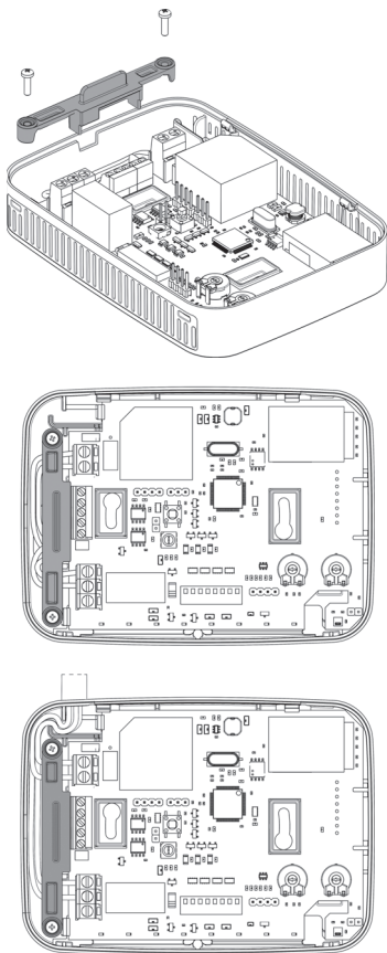
Fig.5: Retención cables / Cable retention / Fissaggio del cavo / Rétention de câbles / Zugentlastung / Kabel borging / Upevnění kabelů
