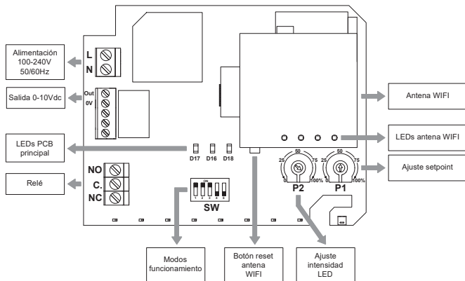
Fig. 1: Placa electrónica
