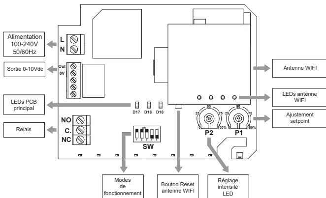
Fig. 1: Plaque électronique
